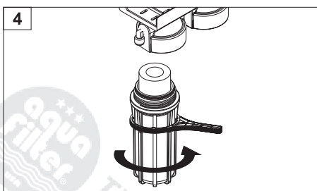
4 Привинтить корпус с картриджем к головке до легкого опора, а потом закрутить до конца, используя ключ. (Помните, чтобы использовать ключ в перпендикулярной плоскости к оси корпуса). Чтобы установить остальные корпуса следуйте соответственно пунктам 1 - 4 инструкции. Внимание! Если не удается довинтить корпус к головке следует проверить правильно ли установлены картриджи и правильно ли расположены уплотнительные кольца.
