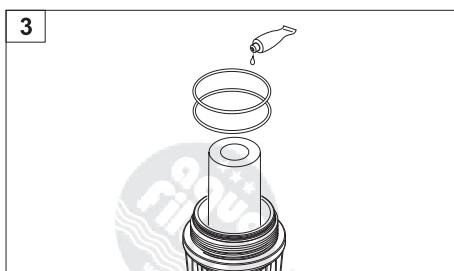
3 Намазать уплотнительные кольца техническим вазелином (отсутствует в комплекте).
