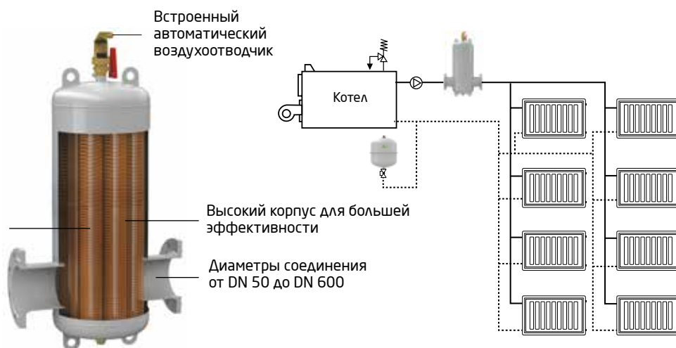
Exvoid HC - пример монтажа
